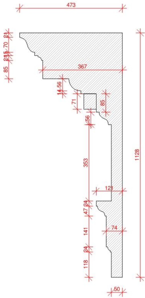
1 PROFILE 1 : 10
