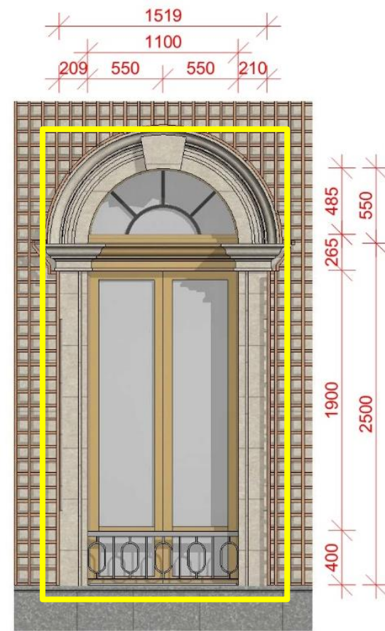
DOOR ELEVATION C
