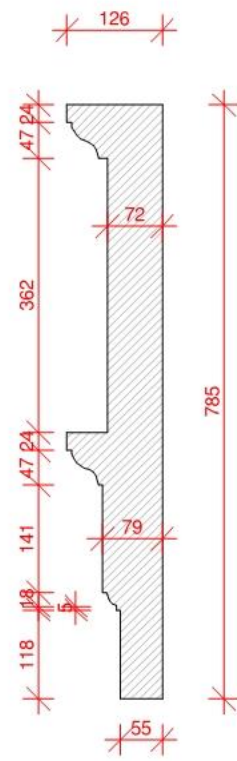
1 PROFILE 1 : 10
